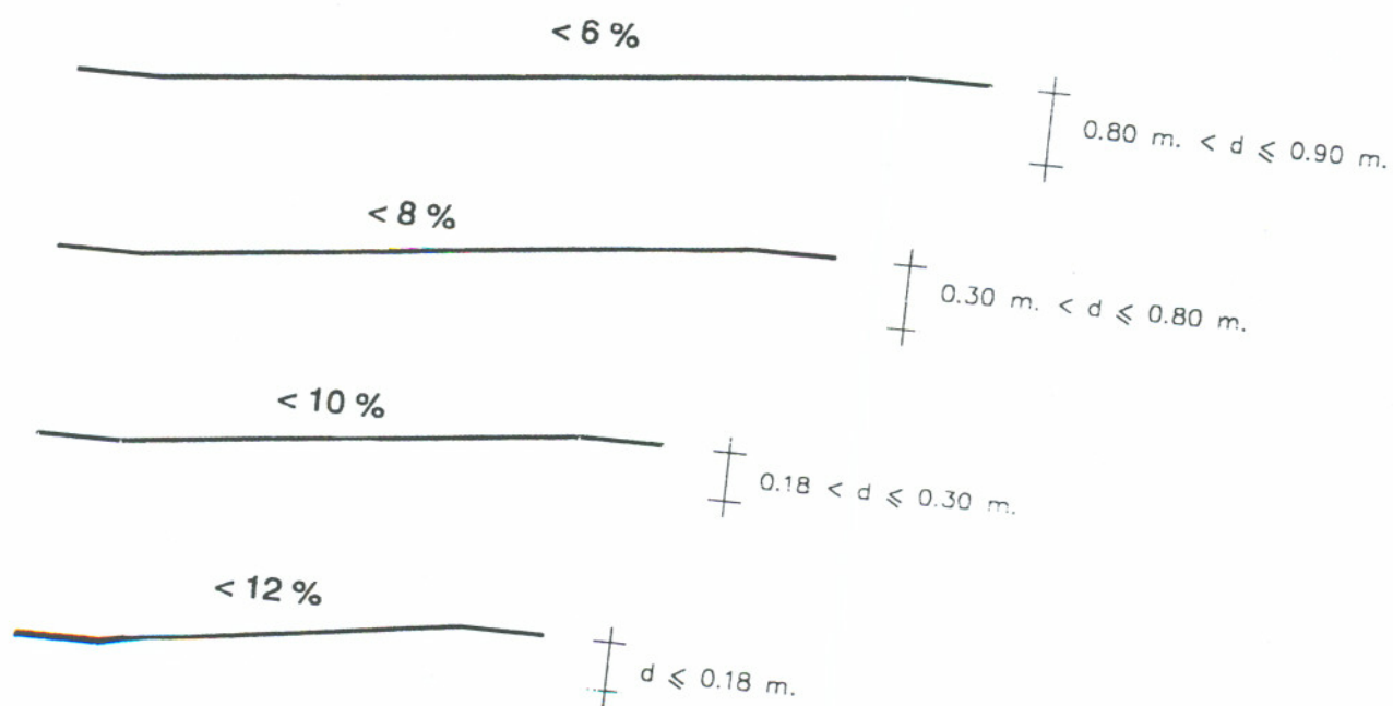
Figura 2. Pendiente longitudinal en función del desnivel
