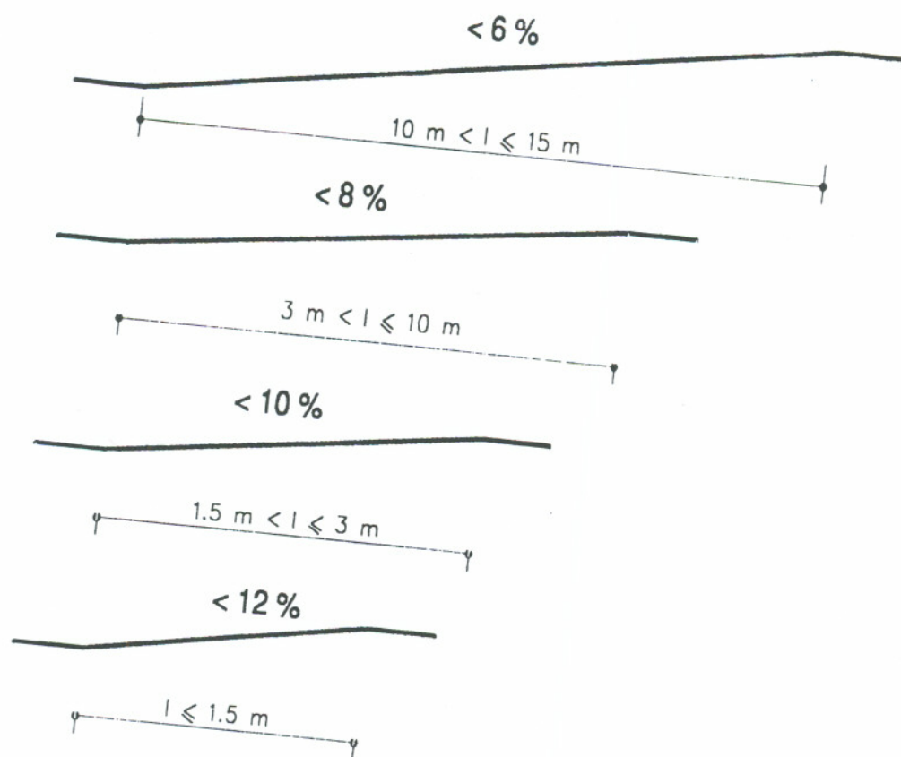
Figura 1. Pendiente longitudinal en función de la extensión
