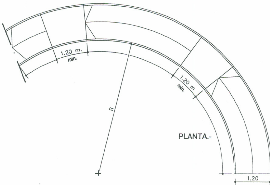
Figura 4. Rampa con cambio de dirección
